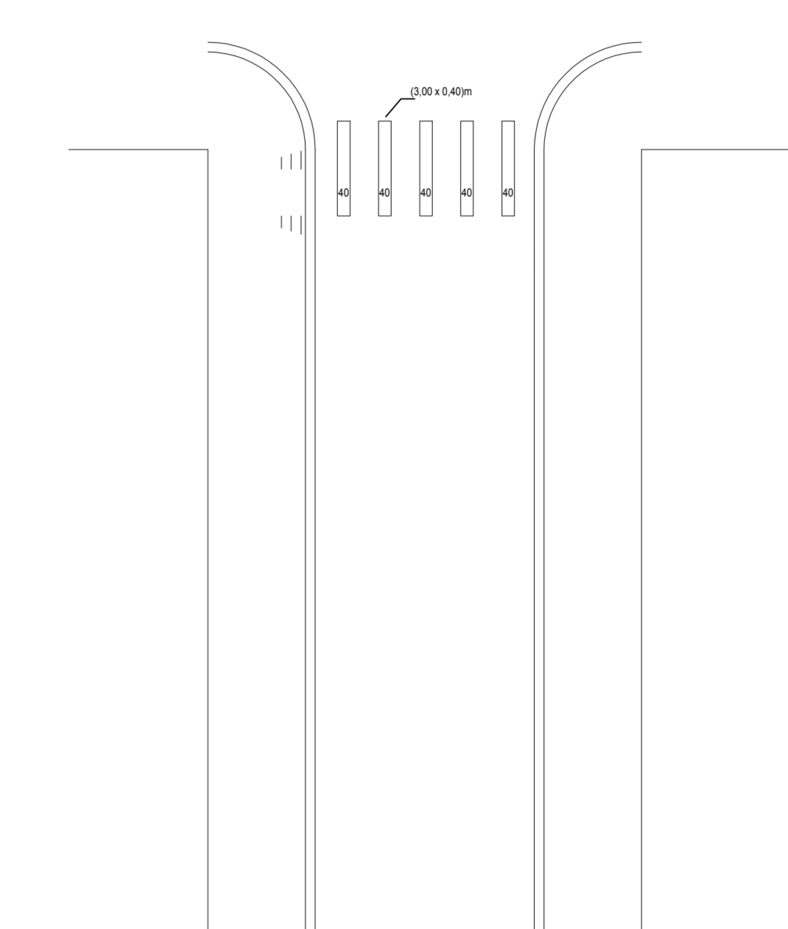
DETALHE DAS FAIXAS 1 LARG. = 6,90m ÁREA = 6,00 m2
