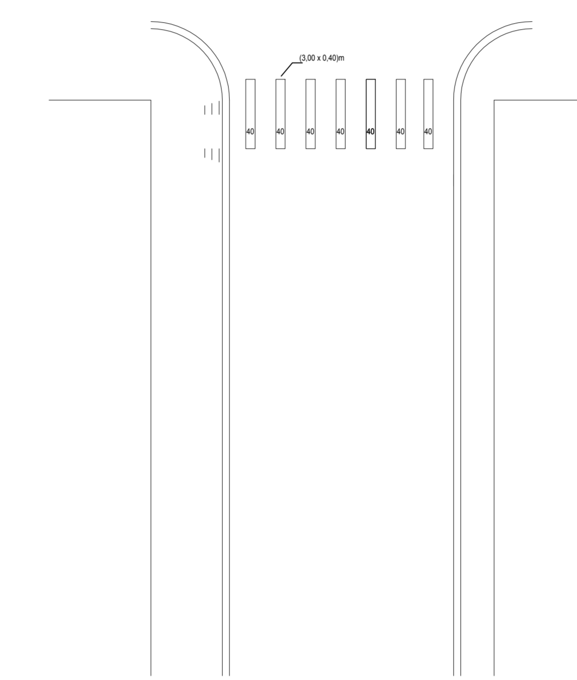
DETALHE DAS FAIXAS 2 LARG. = 8,50m ÁREA = 8,40 m2
