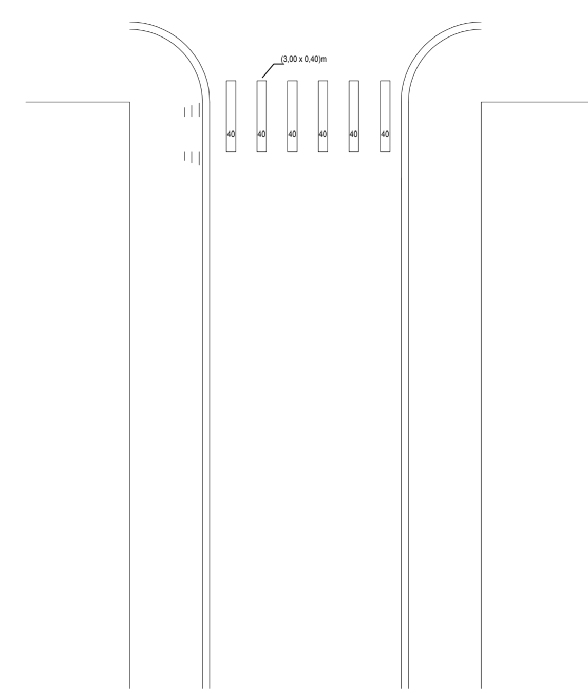
DETALHE DAS FAIXAS 3 LARG. = 7,80m ÁREA = 7,20 m2
